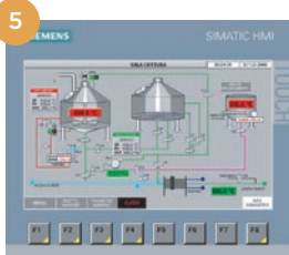
Panel for automatic control of the production process and recipe management. PLC pour la gestion automatique du processus de production et la mémorisation de recettes.
